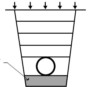
Mise en place non contrôlée
